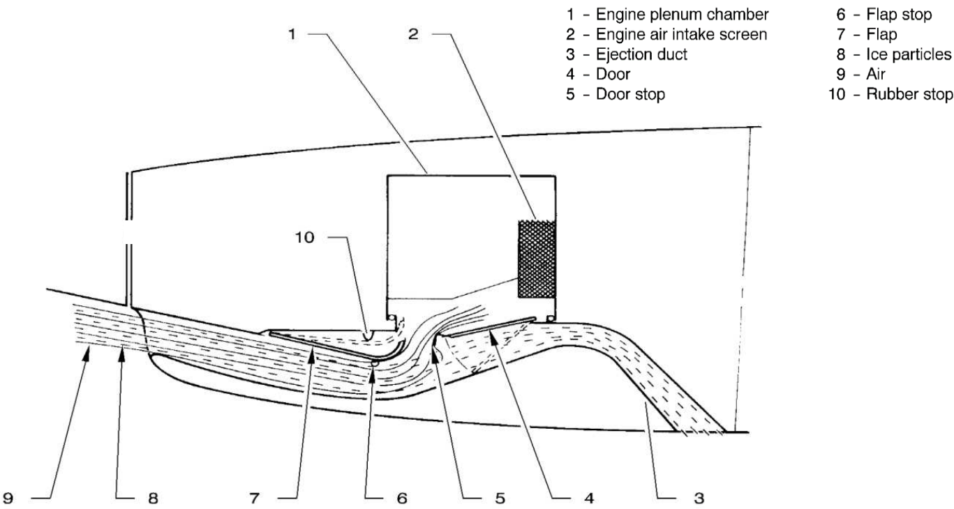
Entrée d'air en position « séparateur activé »
