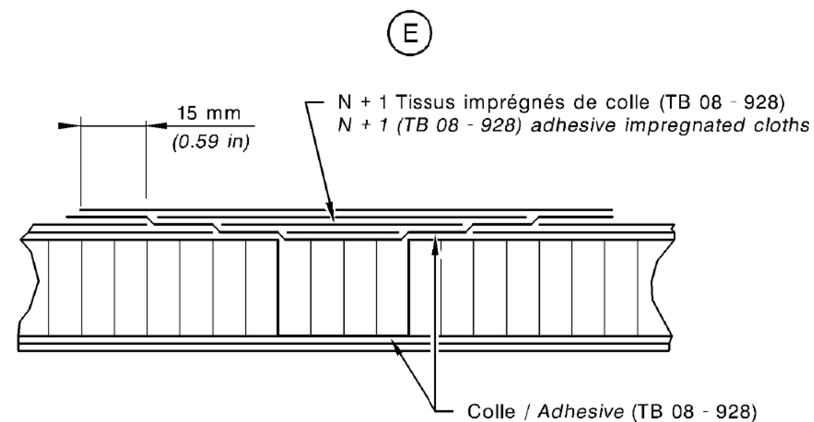
Réparation type 15 BIS Figure 802
