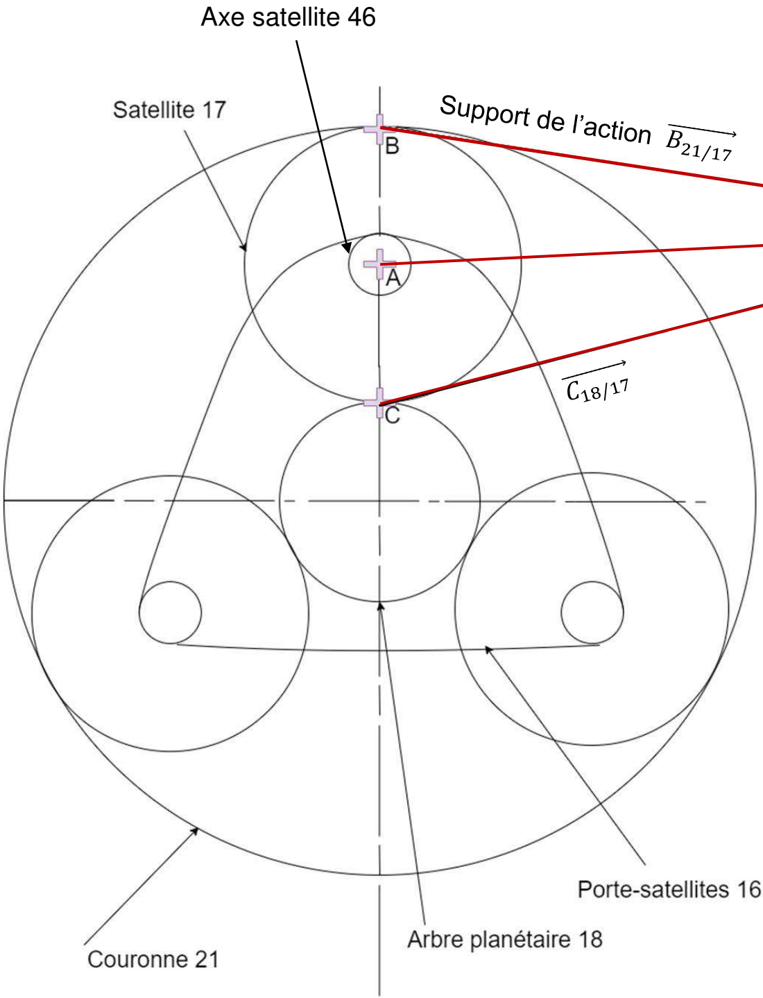
Schéma architectural du 1 er étage de réduction
