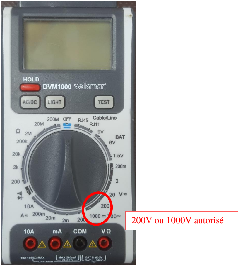
Figure 2 : Multimètre
